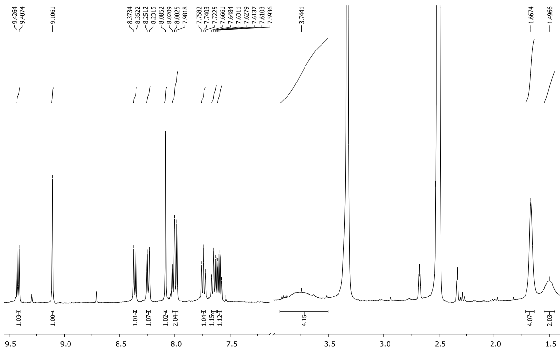
Slika 8. ^1\text{H} NMR spektar benzo[ g ]benzo[4,5]imidazo[1,2- a ][1,8]naftiridin-6-il(piperidin-1-il)metanona 7
