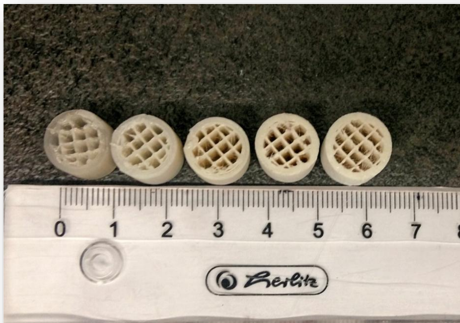
Slika 55. Izrađeni monolitni katalizatori od kompozitnog materijala Z-GLASS + \text{TiO}_2 različitih koncentracija (s lijeva na desno: 0 %, 1 %, 5 %, 7,5 % i 10 %)
