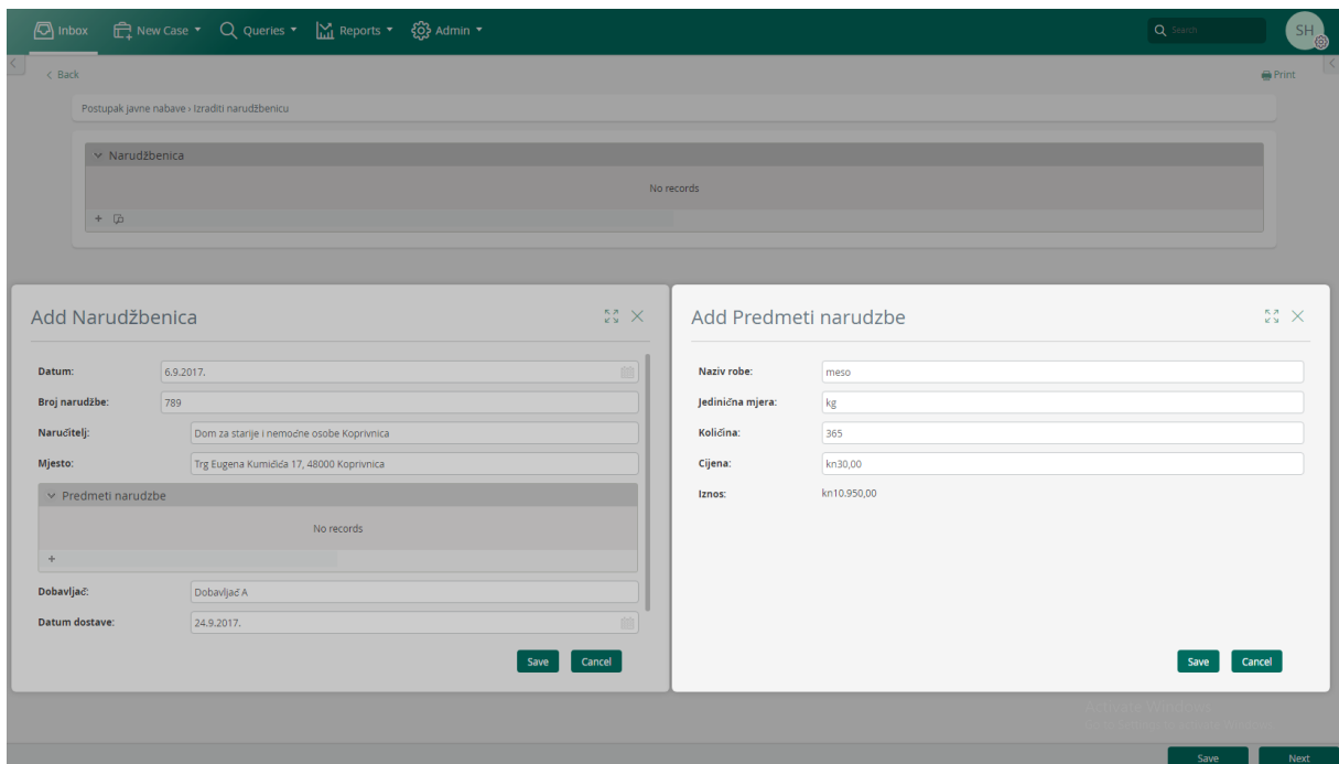
Slika 39 Izraditi narudžbenicu
