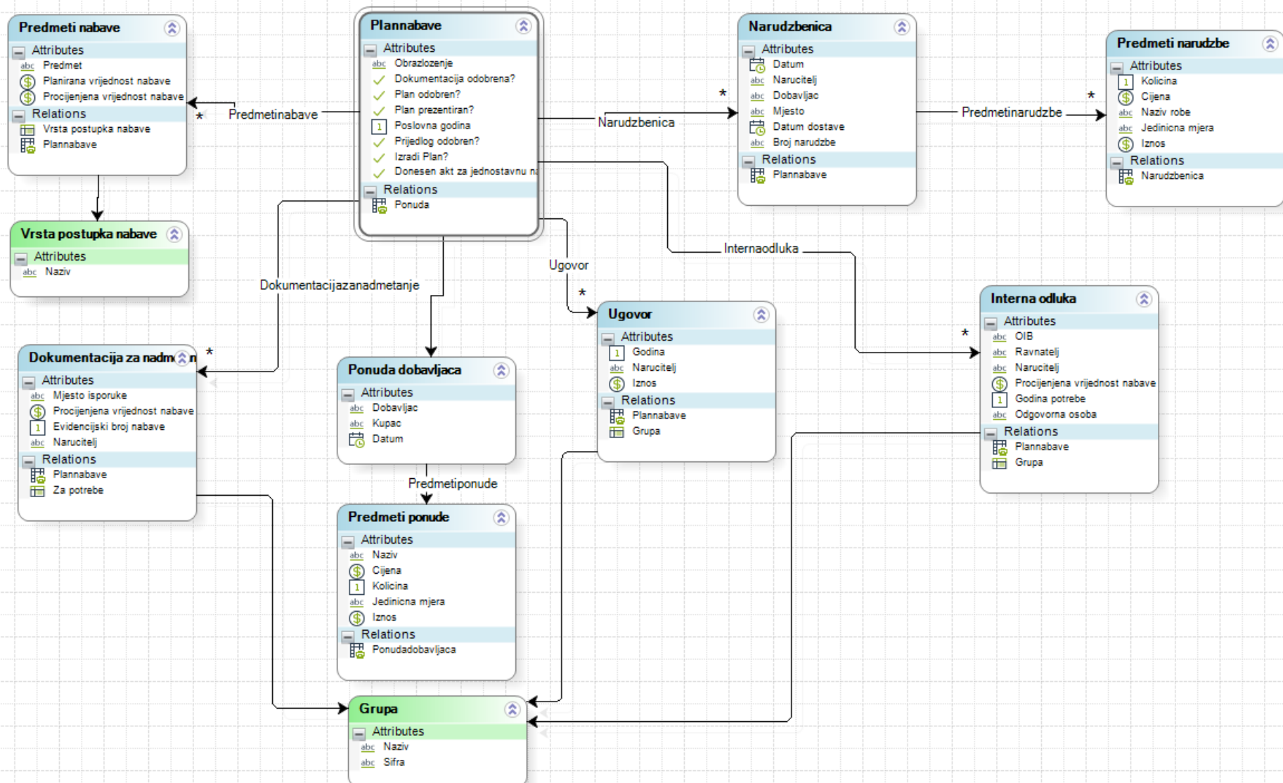
Slika 13 Model podataka
