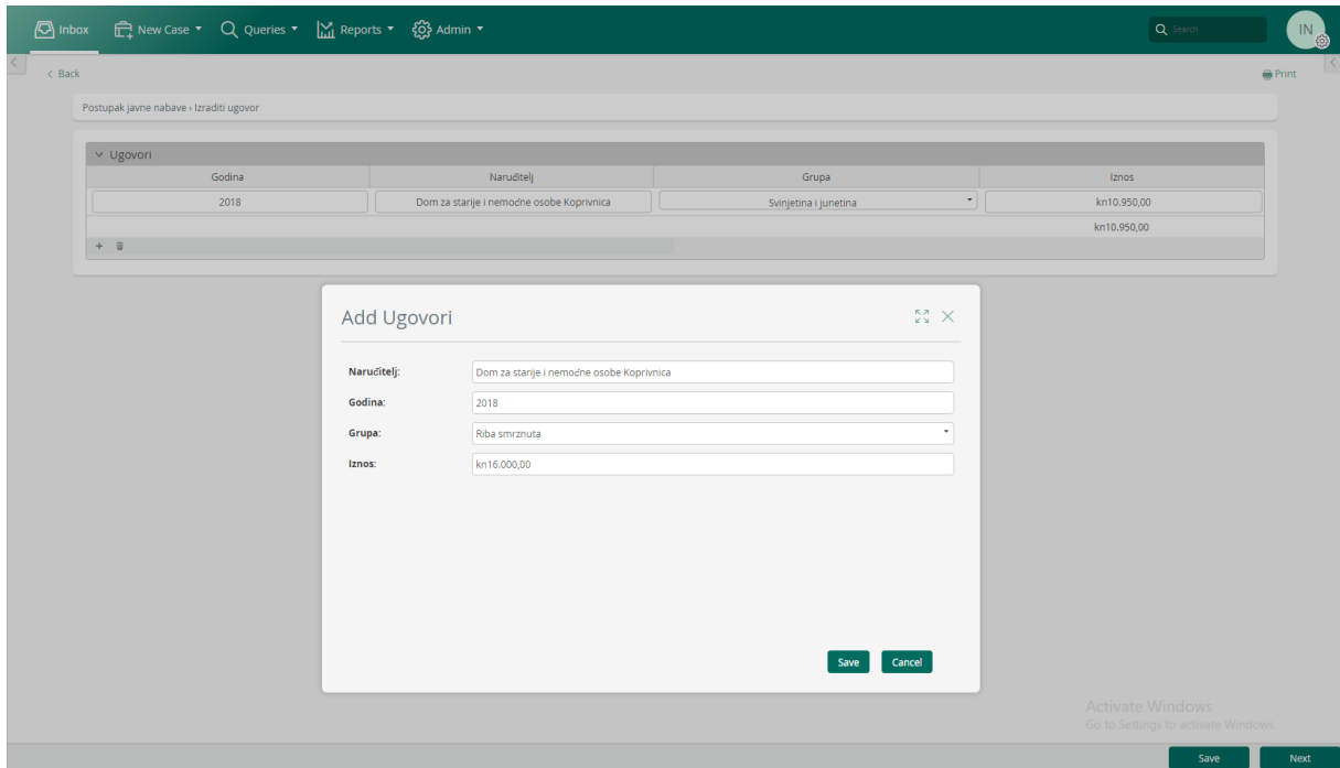
Slika 38 Izraditi ugovor
