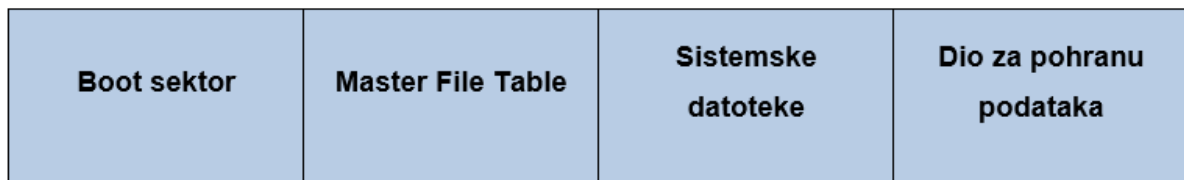
Slika 1. Struktura NTFS-a
