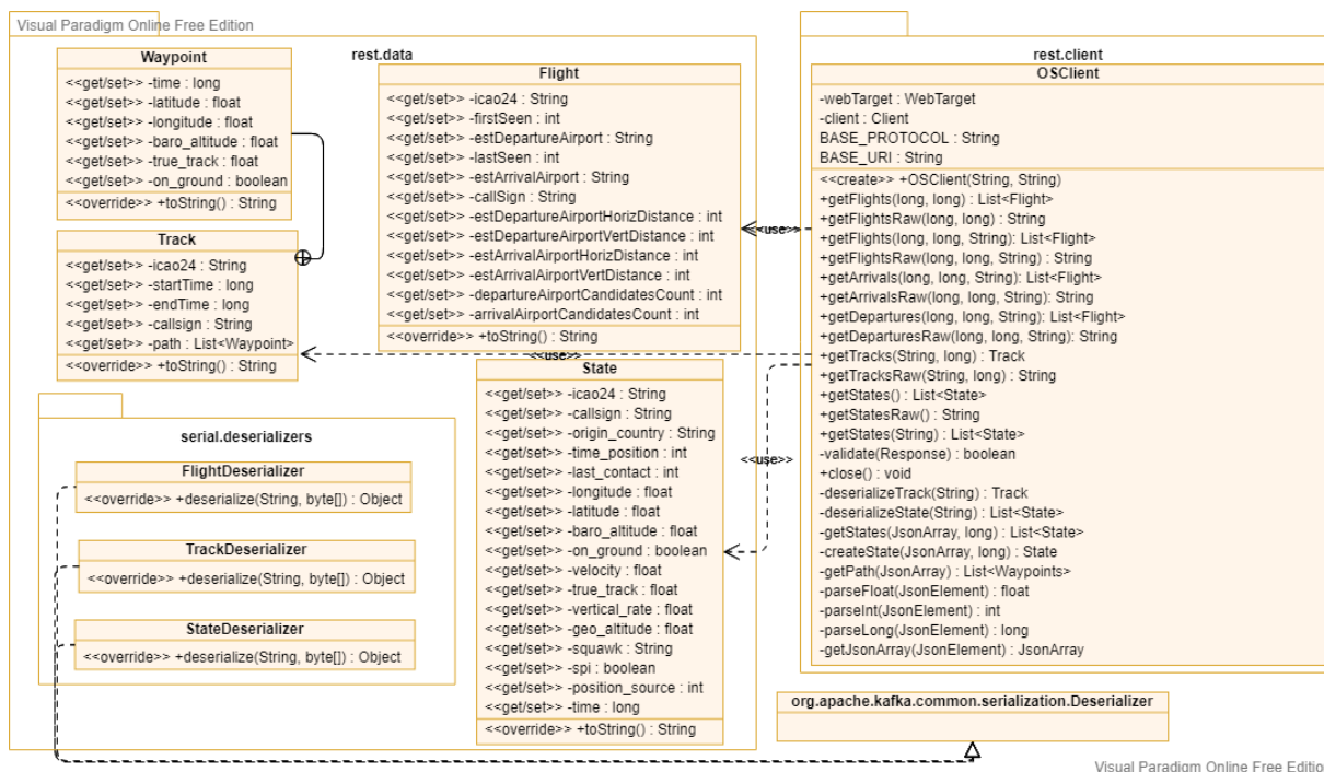
Slika 12: UML dijagram klasa "ilevak_OSNetwork" (Izvor: vlastita izrada)
