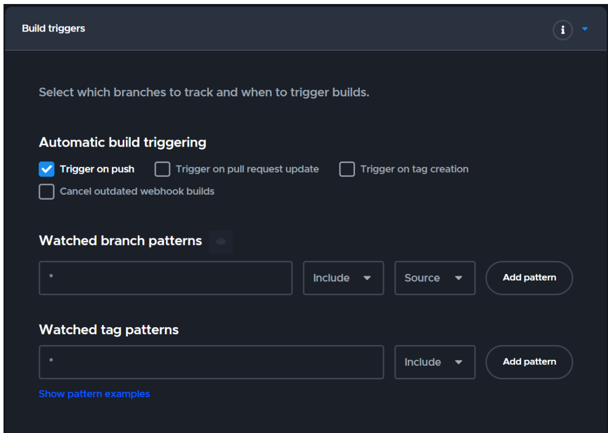
Slika 35: Postavke okidača za automatsku izgradnju i testiranje
