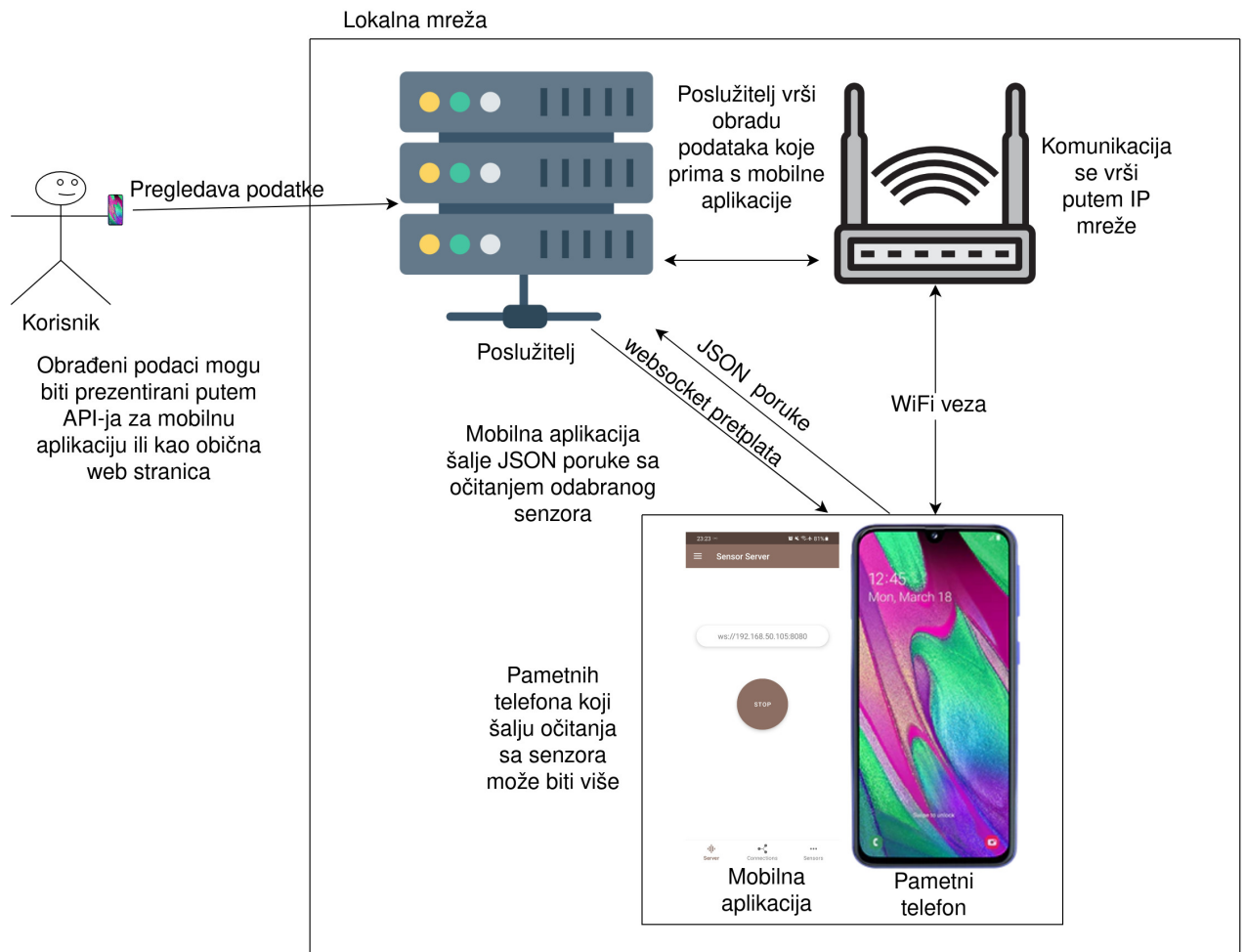
Slika 15 Dijagram - primjer arhitekture M=IoT
