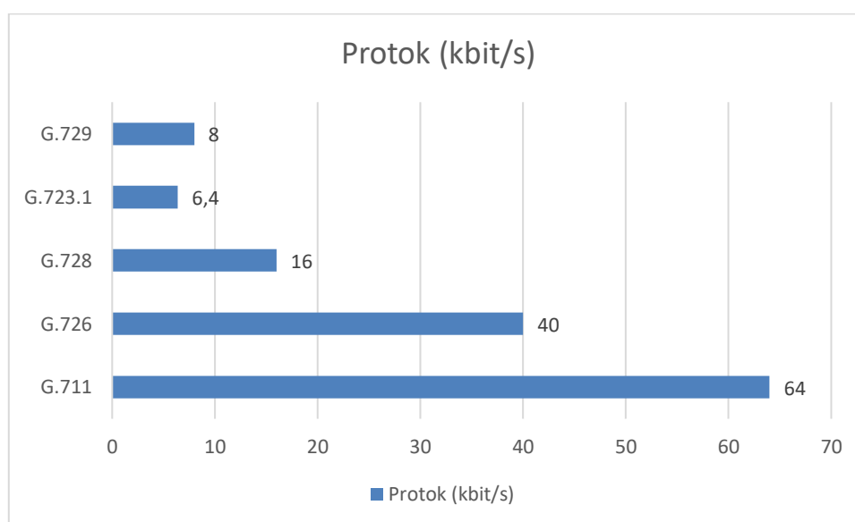
Slika 7. Grafički prikaz protoka korištenih kodeka
