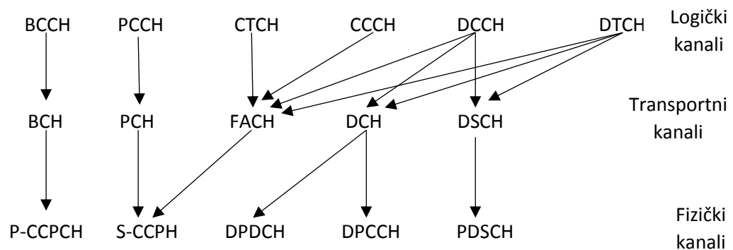
Slika 9. Logički, transportni i fizički kanali u silaznom smjeru veze (bez HSPA), [2]
