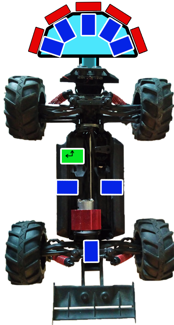
Slika 9: Postava senzora na maketi autonomnog vozila (ljubičasta - infracrveni senzori; crvena - ultrazvučni senzori; zelena - žiroskop)
