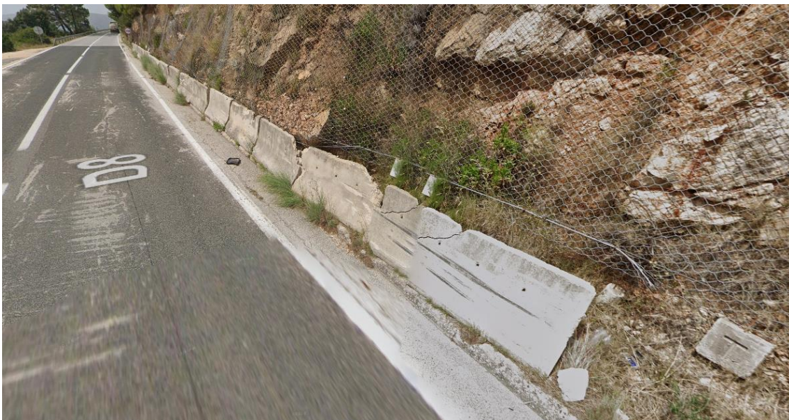
Slika 22. Neadekvatna izvedba betonske zaštitne ograde Izvor:[23]
