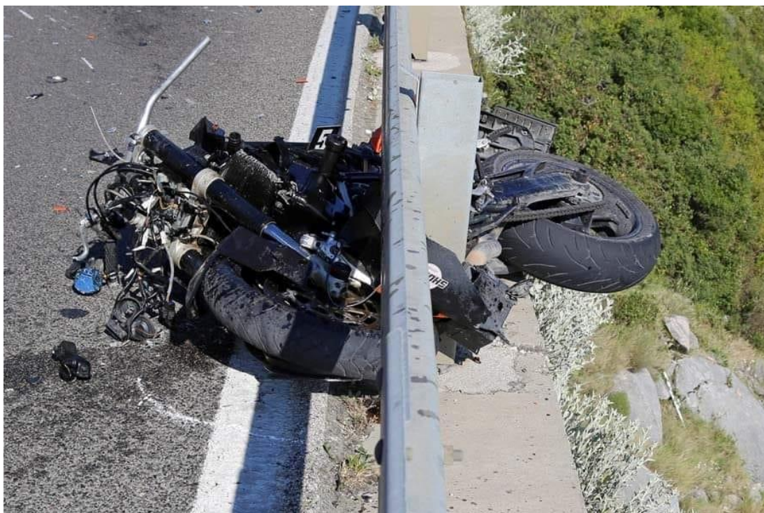
Slika 33. Primjer motocikla koji je podletio pod čeličnu zaštitnu odbojnu ogradu Izvor:[26]
