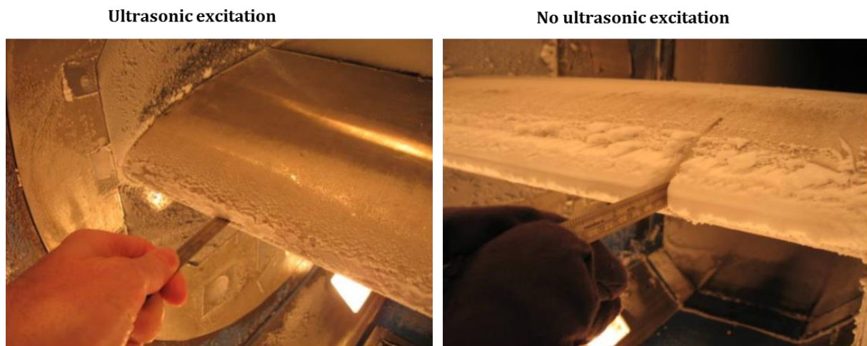
Slika 29. Rezultati provođenja testiranja ultrazvučne tehnologije u zračnim tunelima Izvor: [35]
