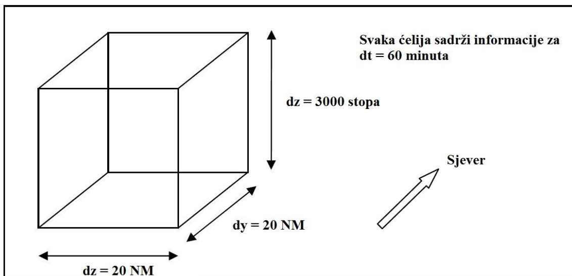
Slika 3 - Dimenzije ćelija
