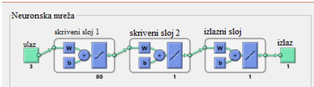
Slika 13: Arhitektura neuronske mreže s dva skrivena sloja
