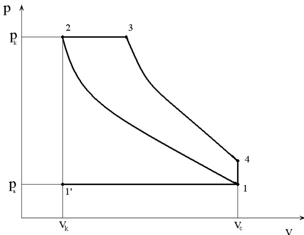
Slika 20. Dijagram teorijskog Dieselova procesa [18]
