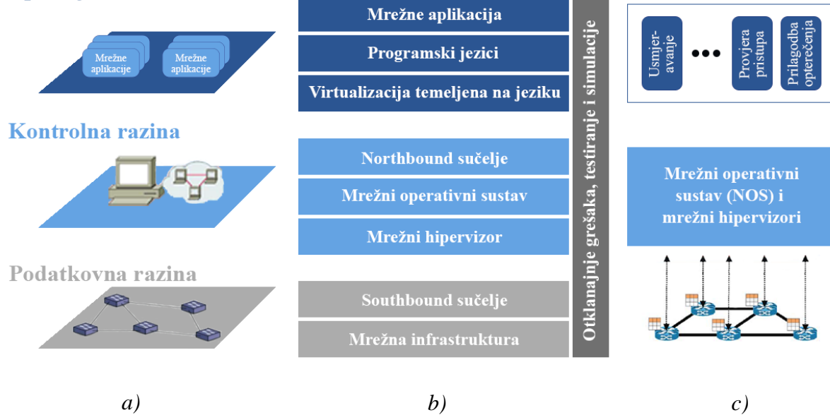
Slika 2 Softverski definirane mreže prikazane kroz: a) razine, b) slojeve i c) arhitekturu dizajna sustava. Izvor: [5]
