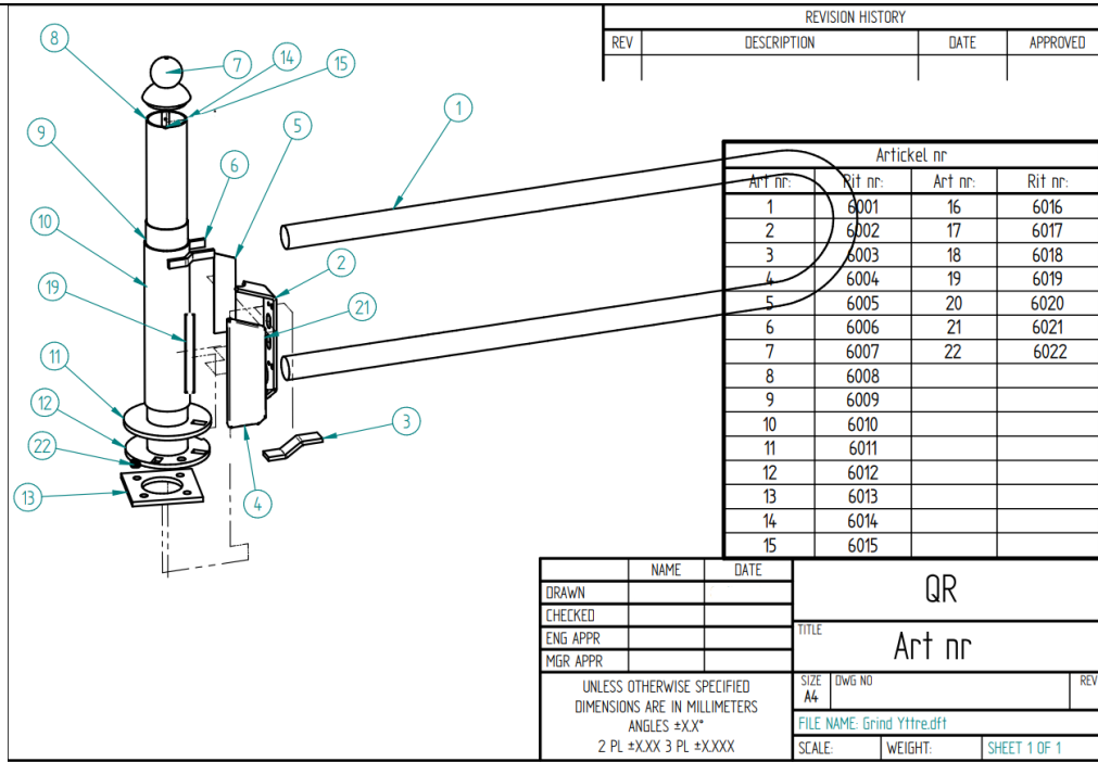
Slika 19. Sklopna sastavnica sa prikazanim dijelovima [9]
