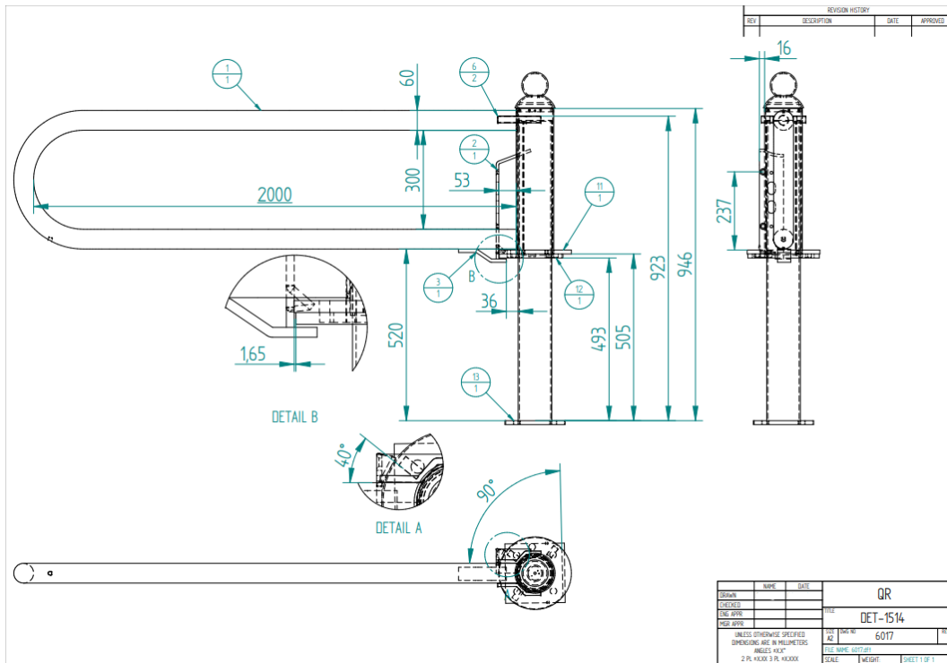
Slika 20. Gabaritne mjere proizvoda [9]
