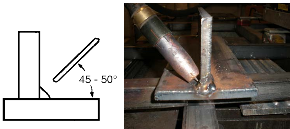
Slika 4.5 Nagib pištolja kod izvođenja kutnog zavara
