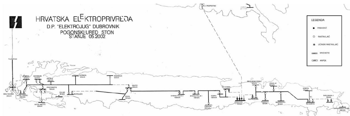
Slika 18. Elektroenergetski sustav otoka Mljeta [5]
