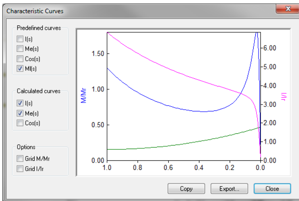
Slika 8. Karakteristična krivulja momenta opterećenja i struje [1]
