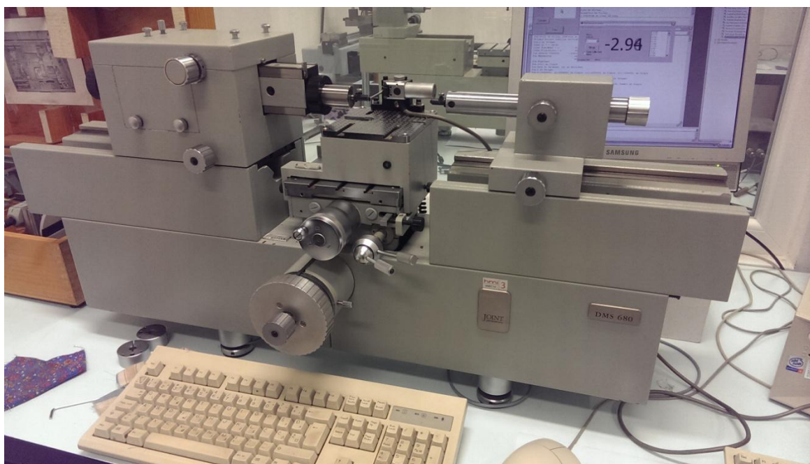
Slika 16. ULM uređaj za umjeravanje ticala
