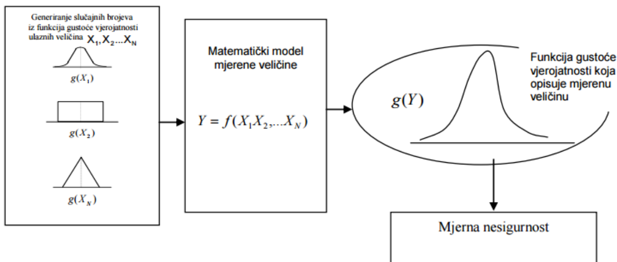
Slika 45. Monte Carlo simulacija mjernog sustava
