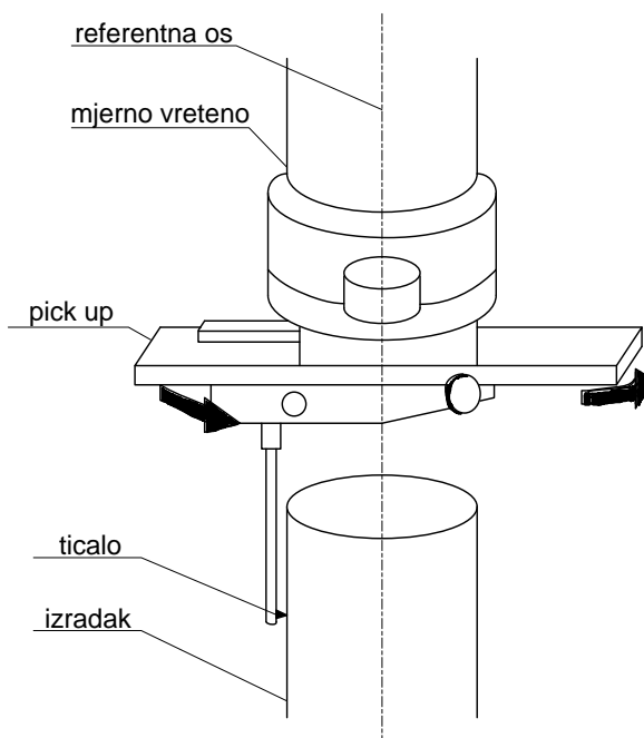
Slika 3. Tip rotirajućeg „pick-up“-a
