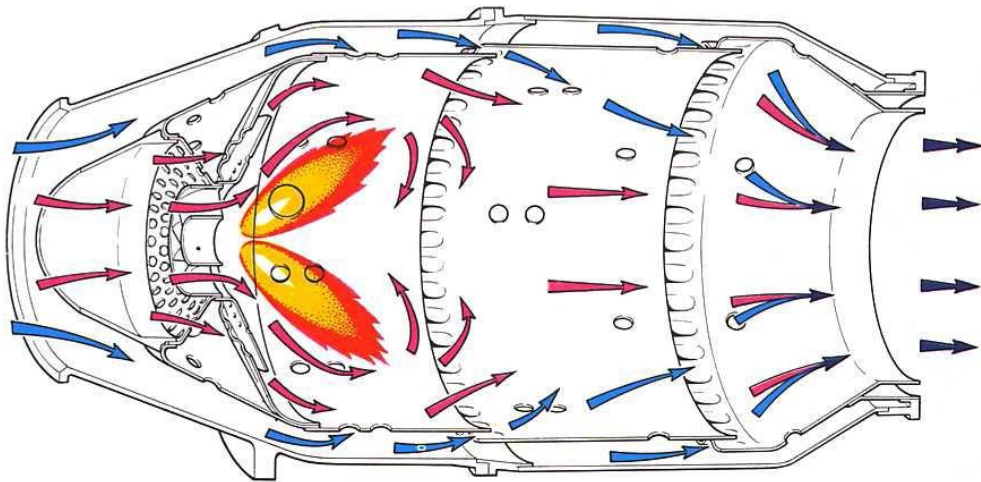
Slika 5. Komora izgaranja [6]
