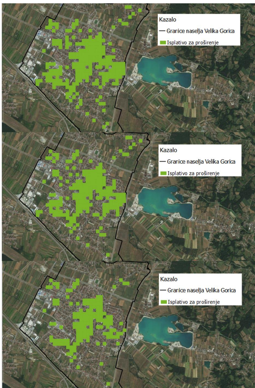
Slika 29 Scenariji 3a, 3b, 3c – Kotao na prirodni plin (stara cijena goriva)
