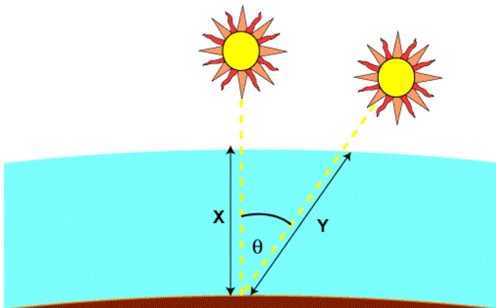
Slika 4. Optička masa zraka
