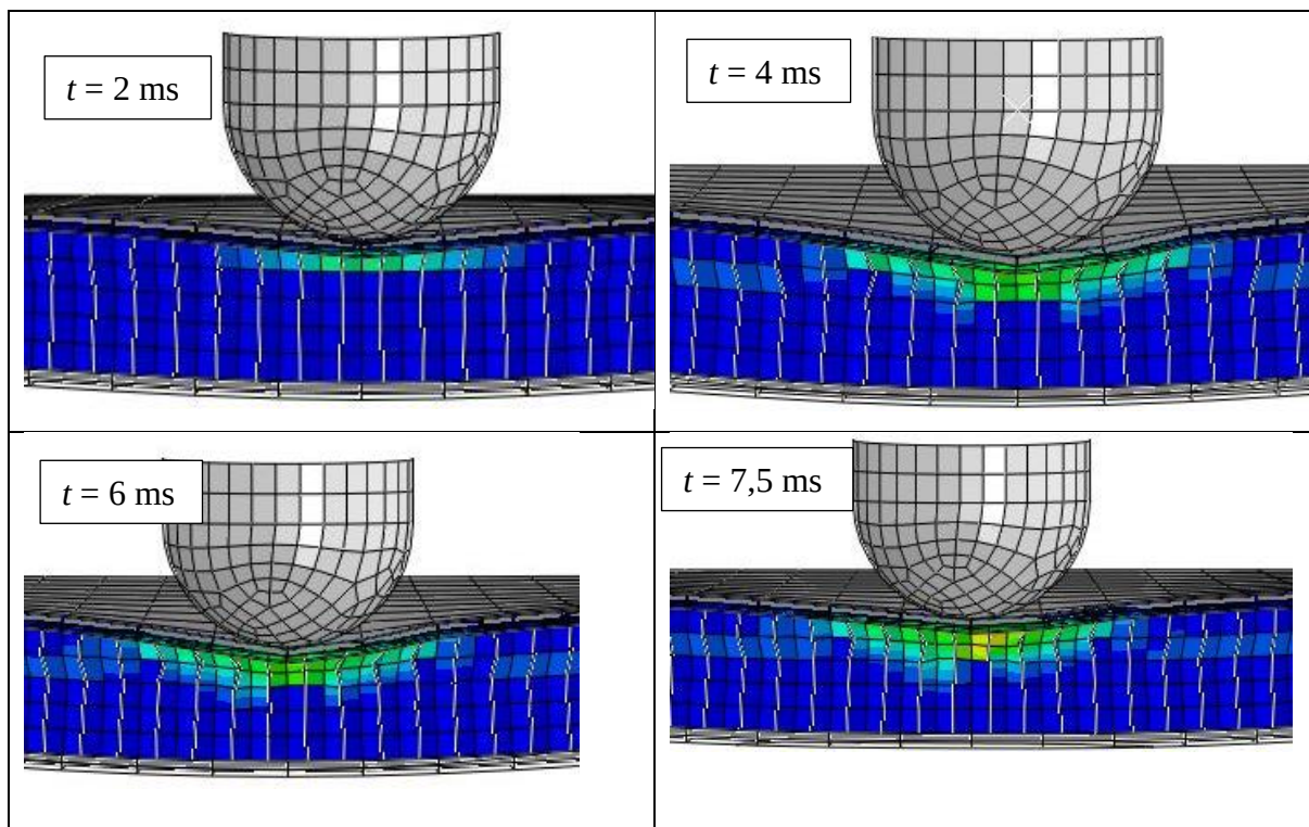
Slika 55: Raspodjela plastične deformacije tijekom trajanja kontakta – sačasti model 0^\circ / 10 J
