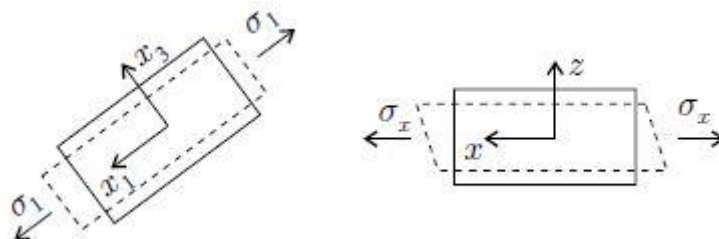
Slika 10: Ortotropni materijal podvrgnut normalnom naprezanju [3]
