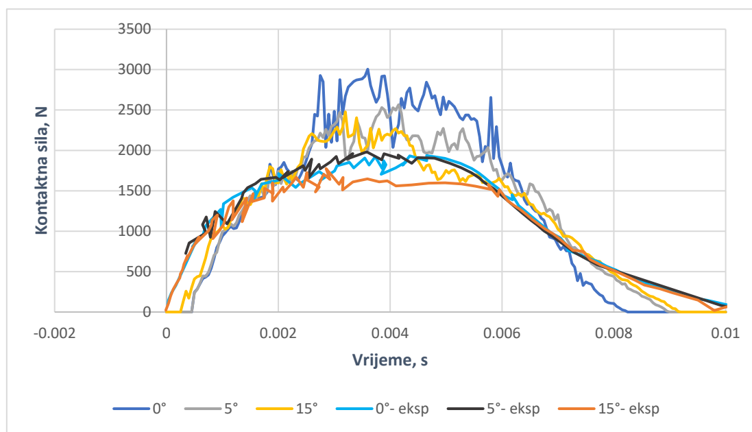
Slika 58: Dijagram kontaktne sile u ovisnosti vremena za energiju udara 10J – sačasti model
