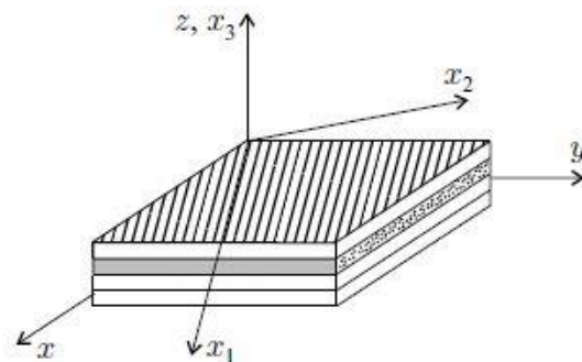
Slika 11: Globalni x, y, z i lokalni x_1, y_1, z_1 koordinatni sustav [3]
