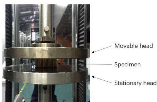
Slika 26: Kvazi-statički test [16]
