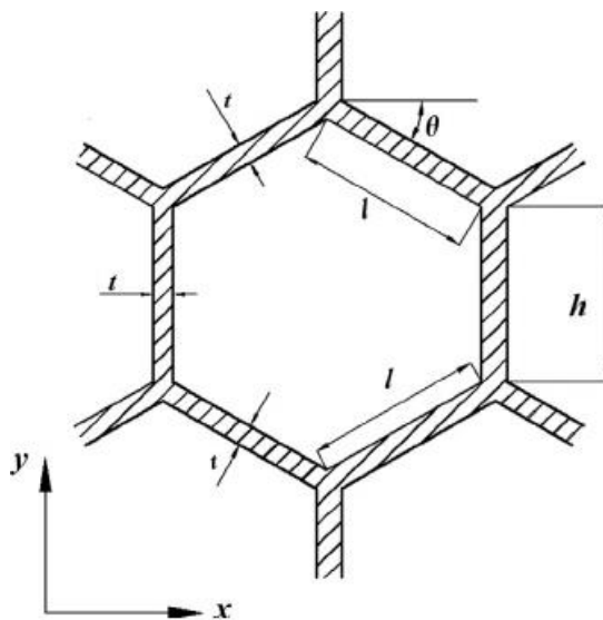
Slika 22: Geometrija saćastih konstrukcija
