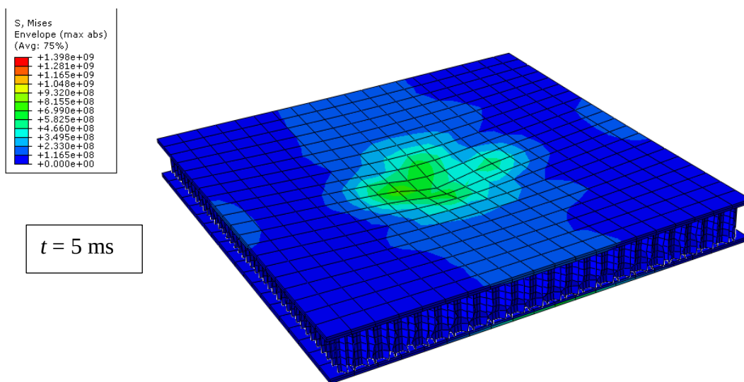
Slika 54: Raspodjela naprezanja po Von Misesu [Pa] za sačasti model za energiju udara 10J i kut udara 0^\circ
