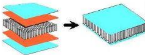
Slika 8: Sandwich paneli [1]
