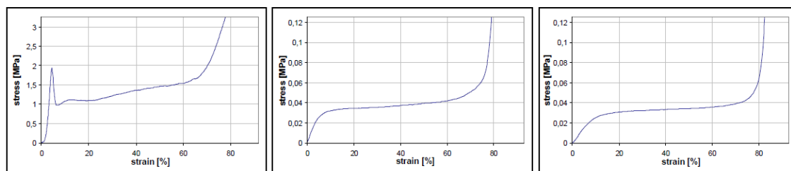
Slika 25: Dijagram naprežanje – istežanje u T, L i W smjeru [14]
