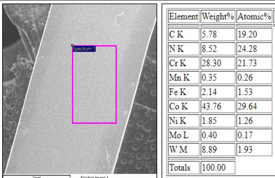
Slika 13. Prikaz lokacije provedene EDS analize s očitanim kvantitativnim sastavom uzorka u nitiranom stanju
