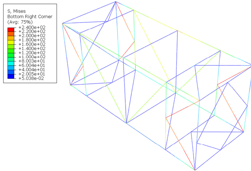
Slika 1. 43 Raspodjela naprezanja prema von Misesu u slučaju opterećenja F=245,7 \text{ Kn}
