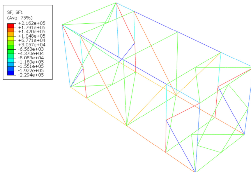
Slika 1. 44 Raspodjela osnih sila pri iznosu sile F=245,7 \text{ kN} .
