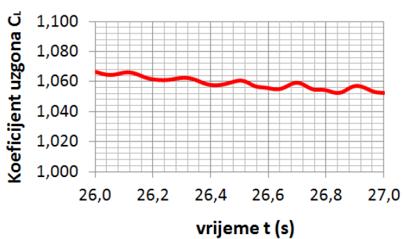
Slika 7.28 C_L pri \alpha=10^\circ (viši red točnosti)
