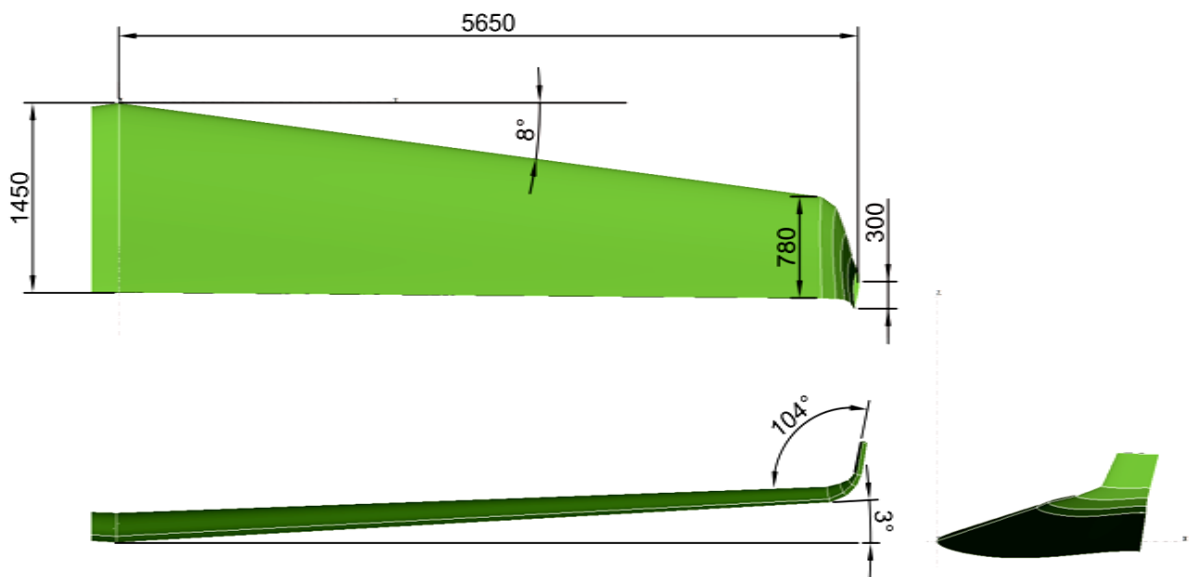
Slika 7.5.4: Nacrt odabranog krila
