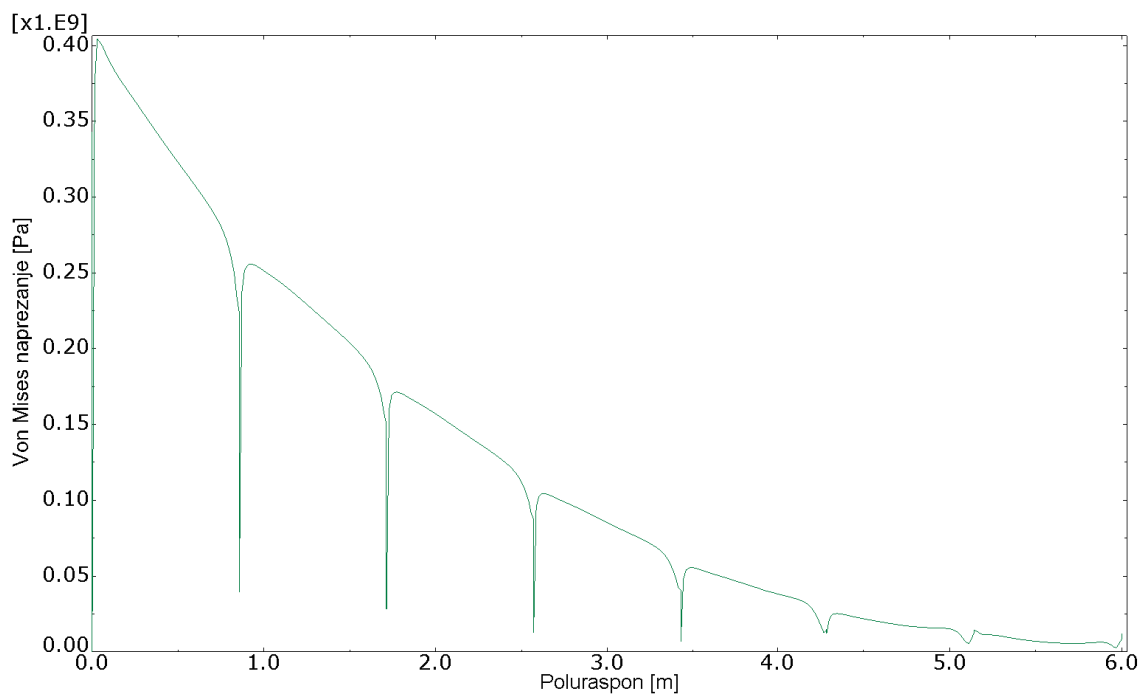
Slika 5.1: Von Misesova naprezanja pri +3 g
