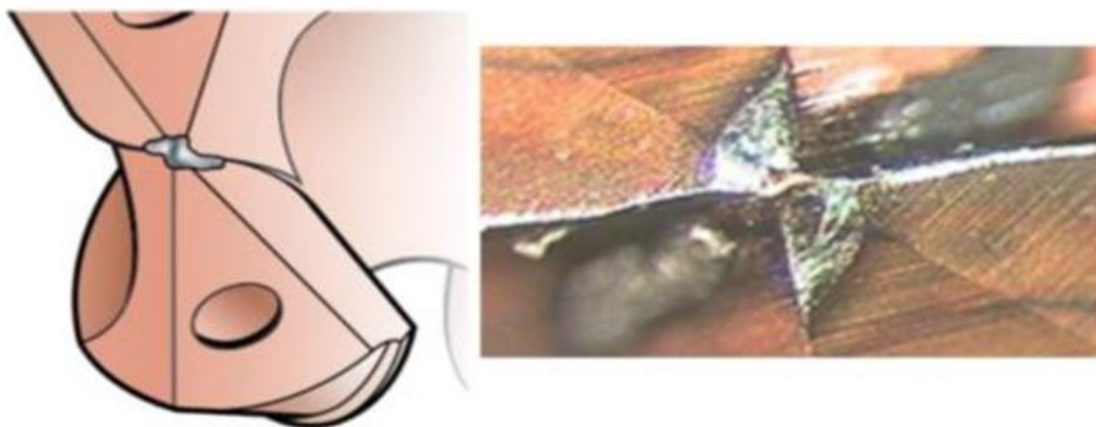
Slika 15. Trošenje stražnje površine poprečne oštrice [12]
