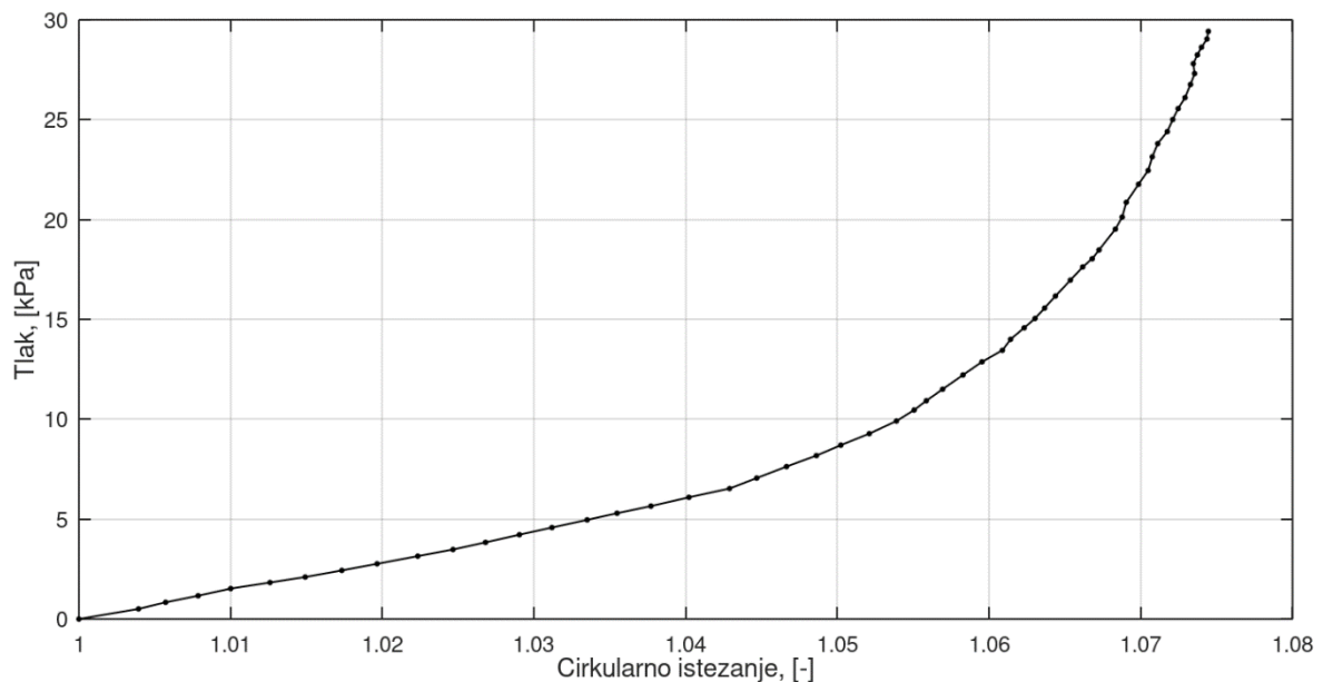
Slika 1.3 - Odziv arterije Donora VIII
