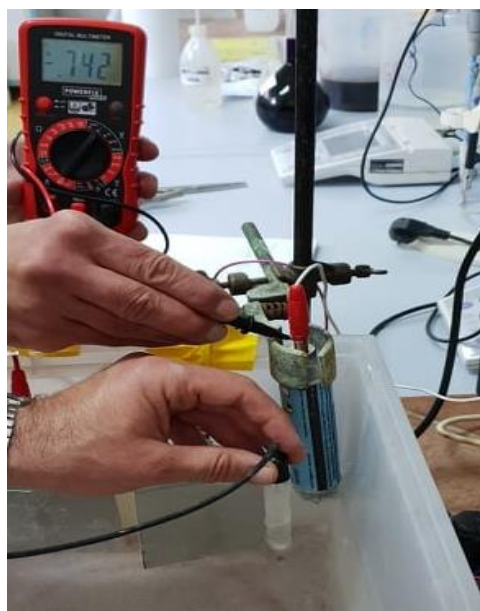
Slika 35. Zasićena kalomel referentna elektroda (lijevo) i prikaz mjerenja (desno) [42]
