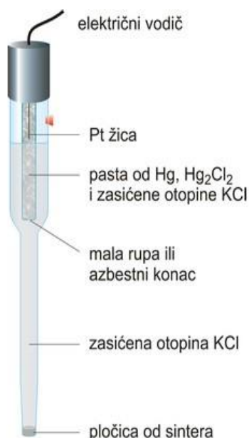
Slika 35. Zasićena kalomel referentna elektroda (lijevo) i prikaz mjerenja (desno) [42]
