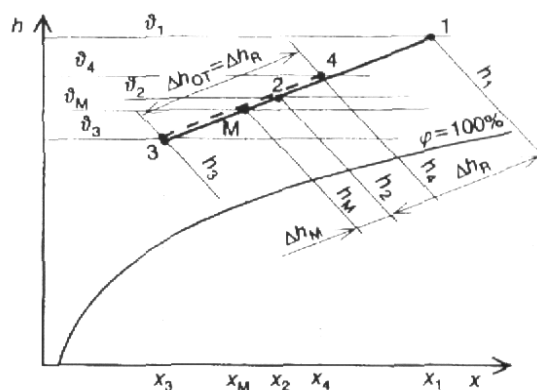
Slika 29. Prikaz procesa u h - x dijagramu, povrat topline sorpcijskim rotacijskim regeneratorskim – ljetno razdoblje
