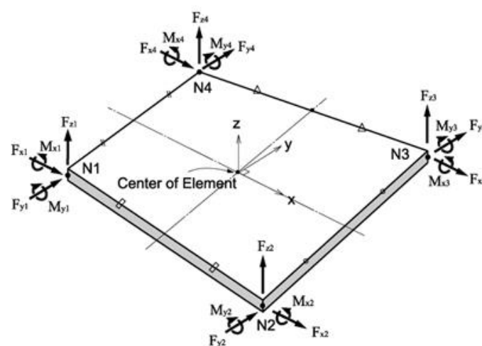
Slika 2. Prikaz pločastog konačnog elementa [8]
