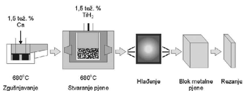
Slika 3.3. Proces nastajanja metalne pjene ALPORAS metodom [4]
