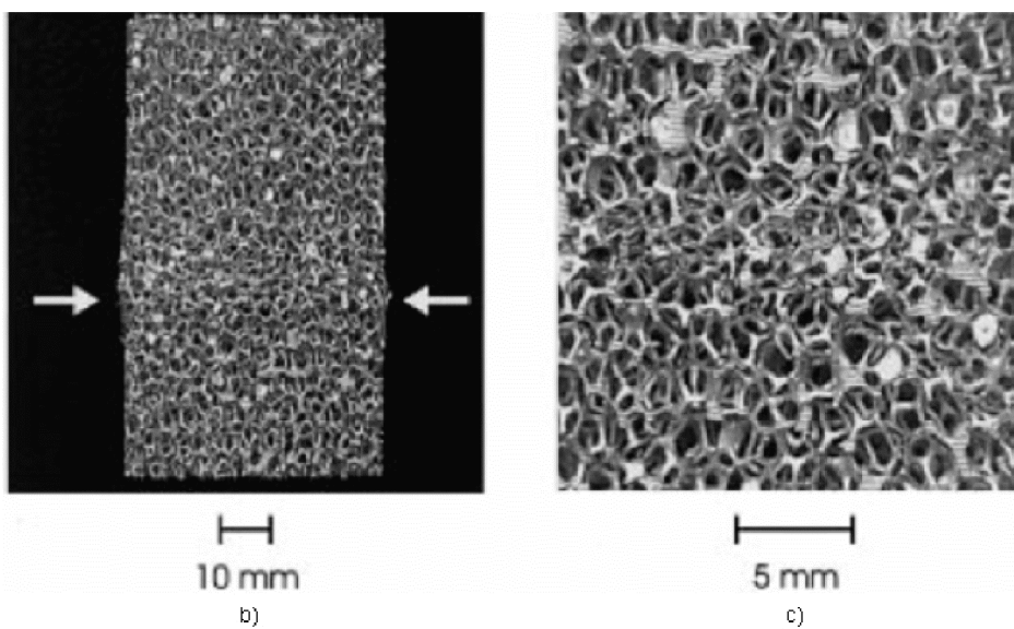
Slika 5.20. d) Lom Al-pjene otvorenih ćelija uzrokovan vlačnim opterećenjem e) Pojasno zadebljanje zbog tlačnog opterećenja f) Pojasno zadebljanje zbog tlačnog opterećenja (uvećani prikaz)[7]
