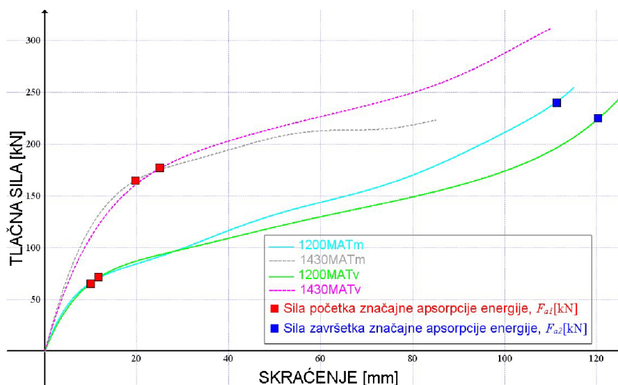
Slika 6.26. Dijagram TLAČNA SILA – SKRAĆENJE za srednje krivulje svih skupina uzoraka.
