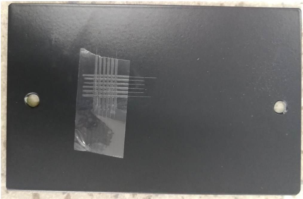
Slika 35. Ljepljenje trake na mrežu nakon zarezivanja prevlake
