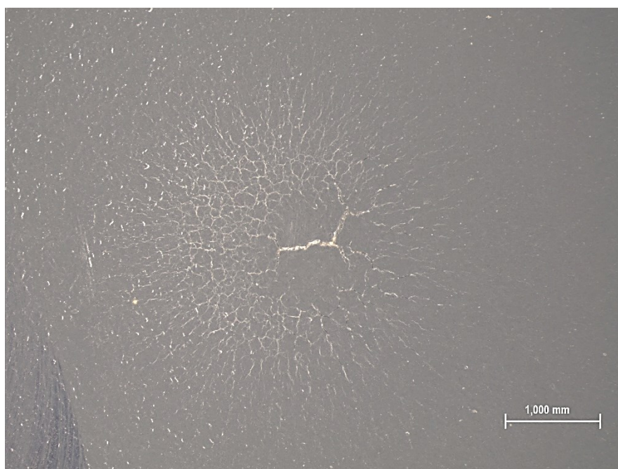
Slika 59. Uzorak N3 - ne zadovoljava; visina s koje je pušten uteg pri kojoj prevlaka nije zadržala svoja svojstva kao ni mikro i makro konzistentnost iznosi 5 cm
