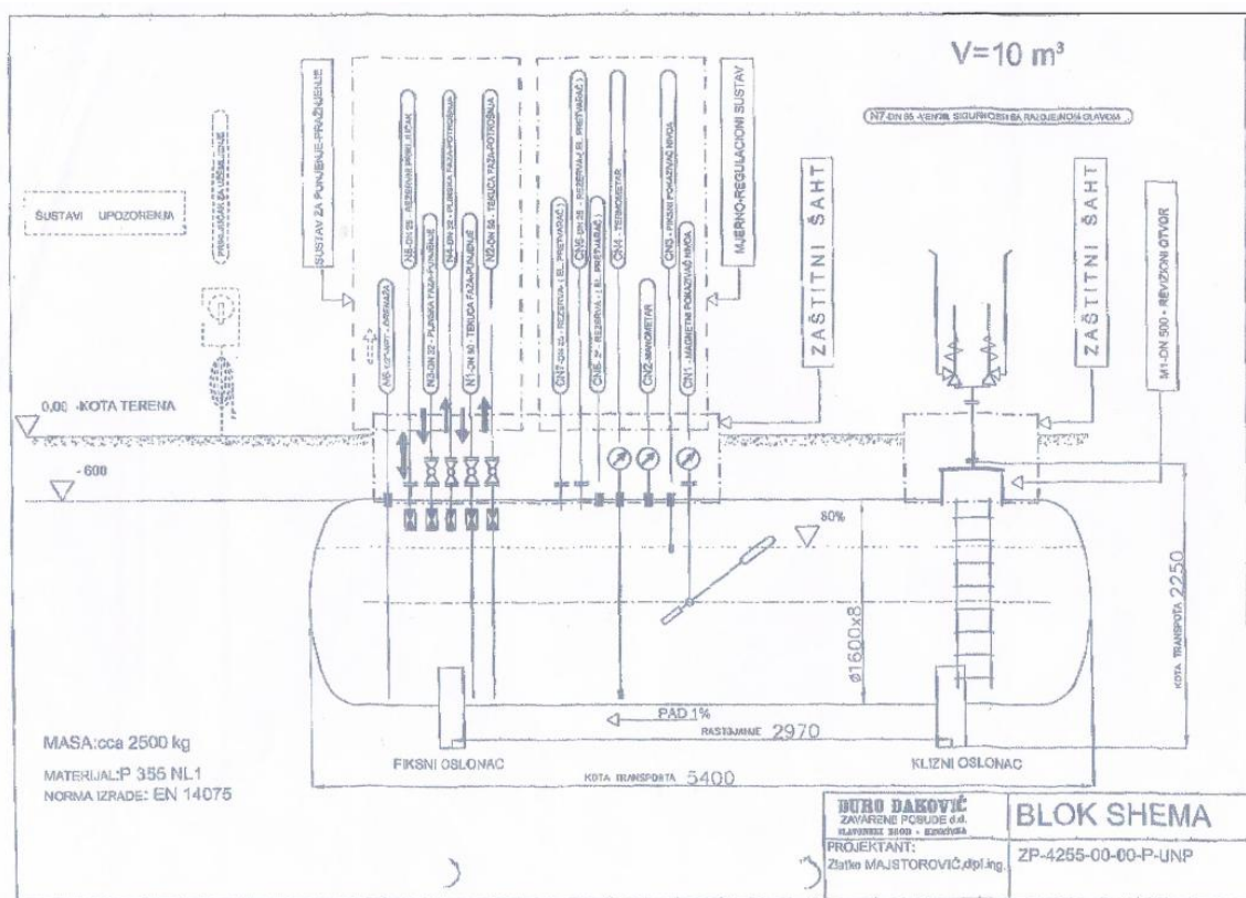
Slika 5. Blok shema spremnika za UNP volumena 10\text{ m}^3 , Đuro Đaković- Zavarene posude
