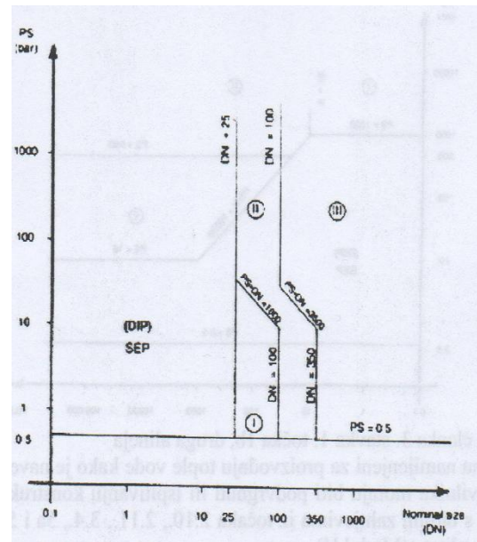
Dijagram 6. Cjevovodi za plinove grupe 1
