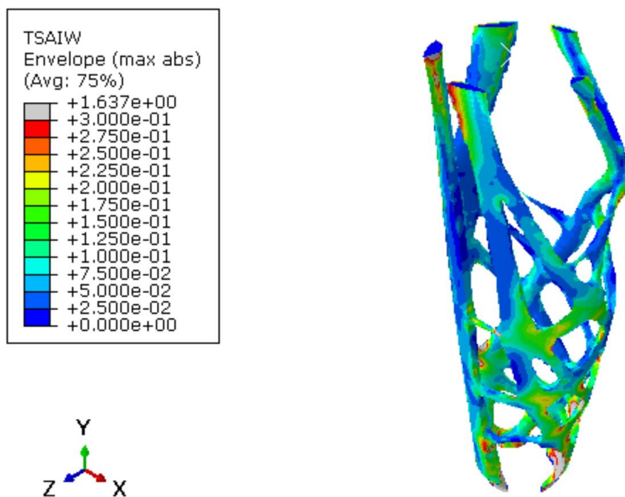
Orijentacija vlakana 0°
