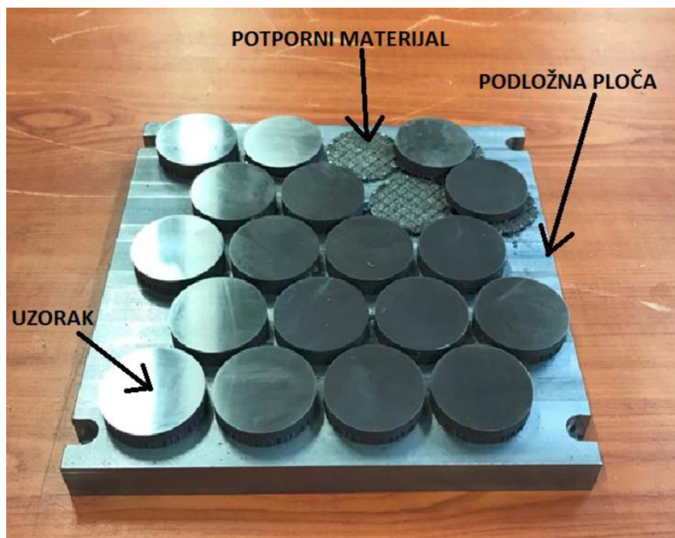
Slika 17. Uzorci napravljeni SLM postupkom na EOS M 290 uređaju
