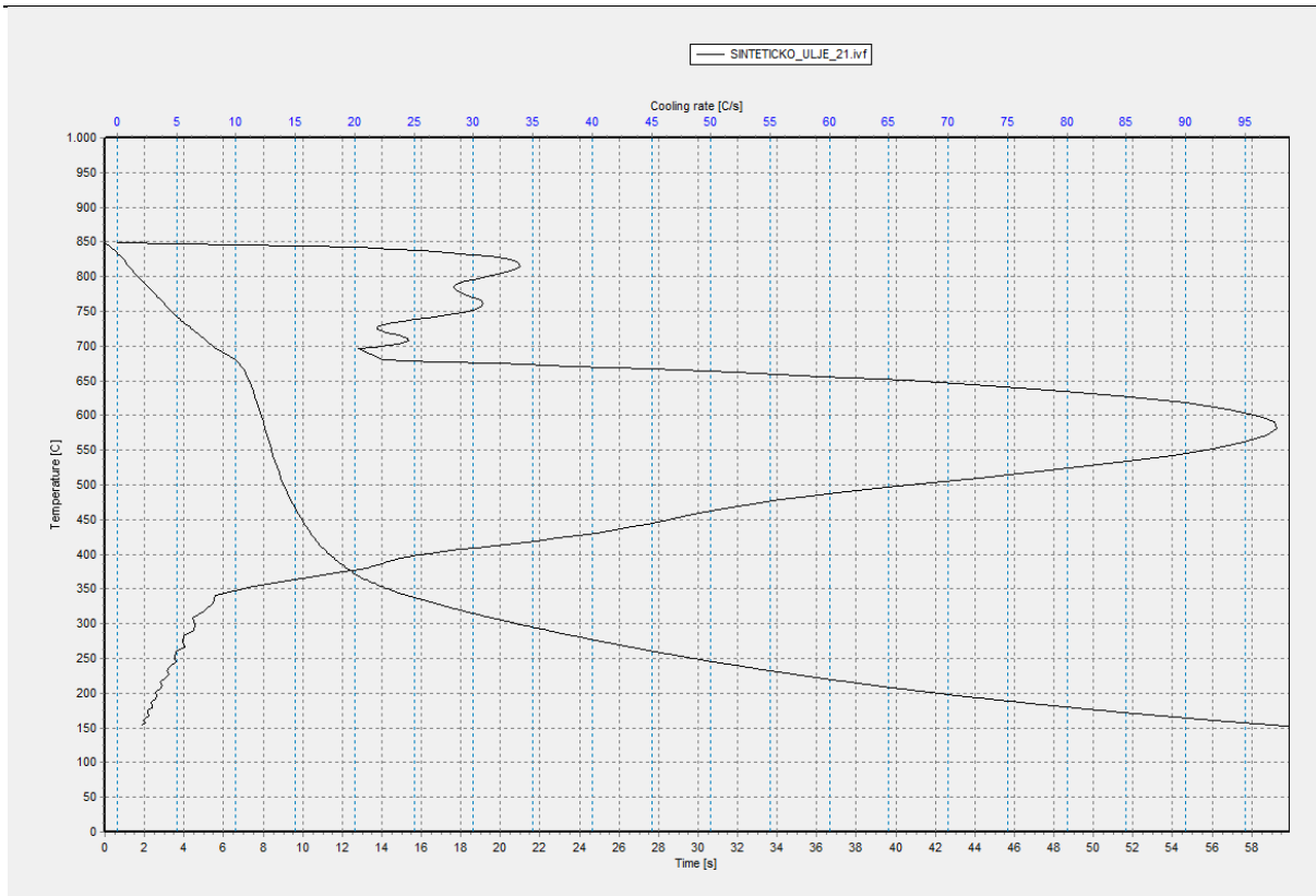
Slika 17. Krivulja ohladijanja (temperatura-vrijeme) i krivulja brzine ohladijanja (brzina ohladijanja-temperatura) ispitnog uzorka sredstva za kaljenje oznake SINTETICKO_ULJE_21
