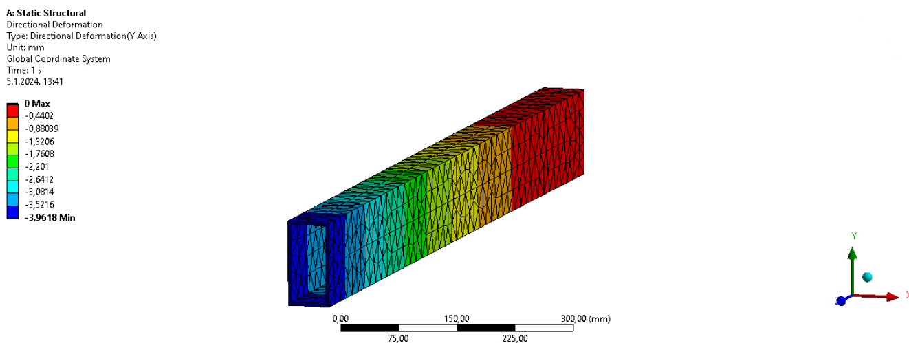
Slika 28. Raspodjela pomaka u mm u smjeru y s tetraedarskim elementima
