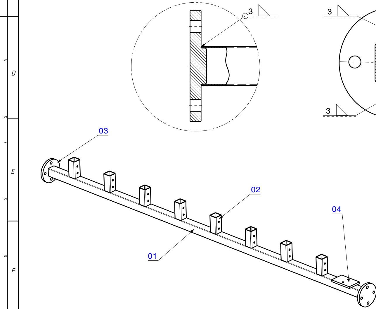
Detalj B M1:2
