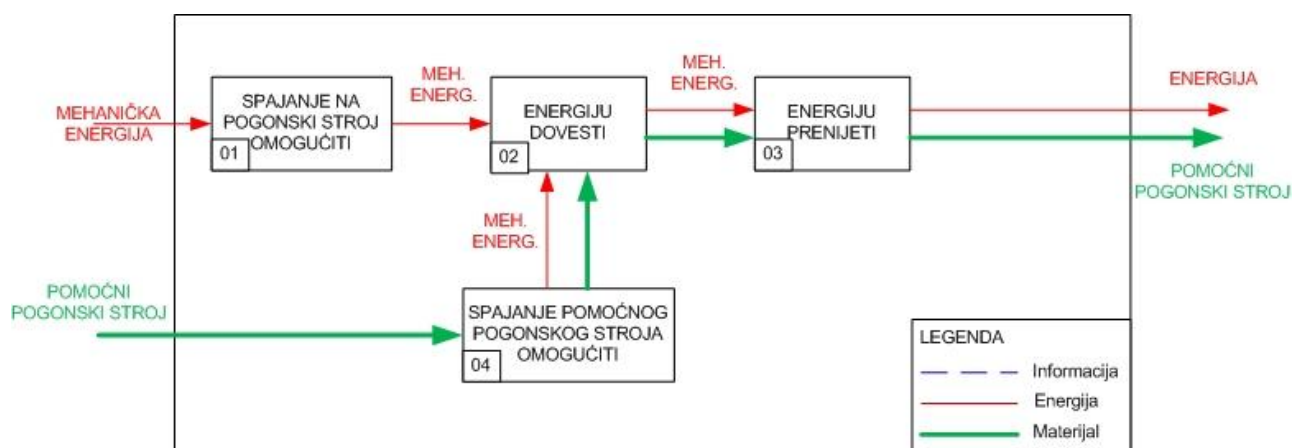
Slika 4.2. Podgrupa P1 funkcijske strukture
