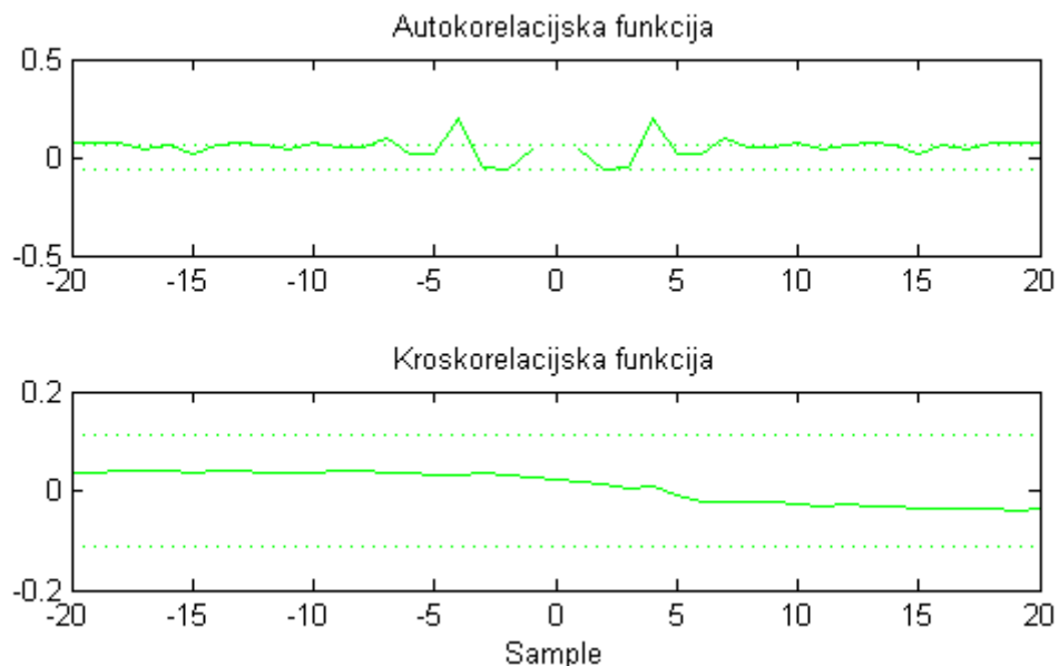
Slika 43. Autokorelacijska i kroskorelacijska funkcija – PRMS
