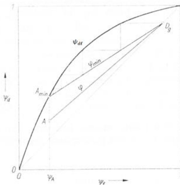
Slika 16. Minimalni refluks [1]
