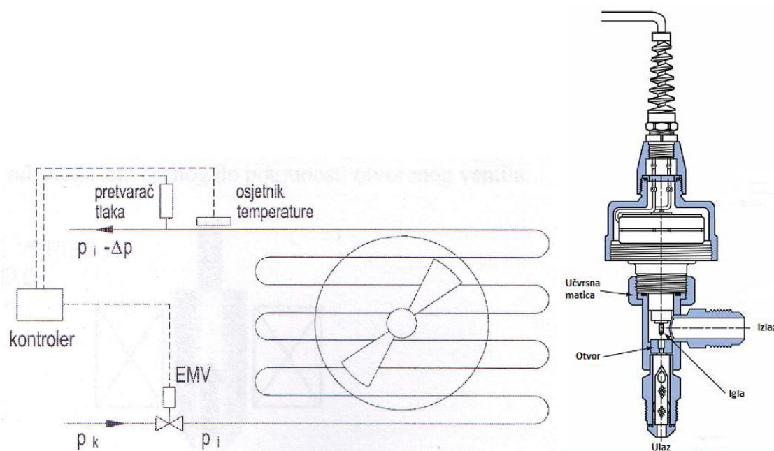
Slika 14. Shema postavljenja EEV-a [5] i EEV u presjeku [11]
