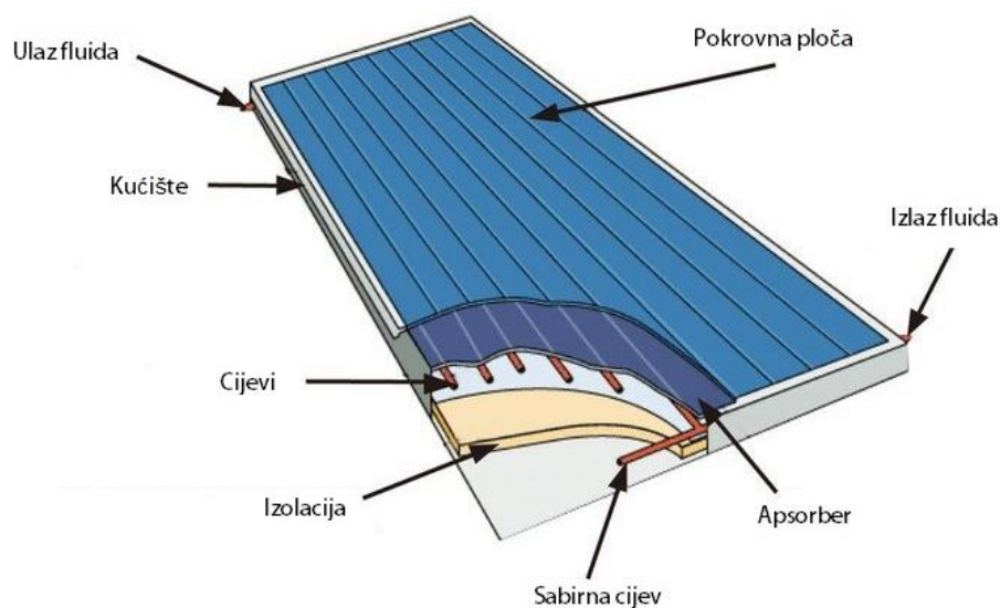
Slika 3. Pločasti solarni kolektor [5]
