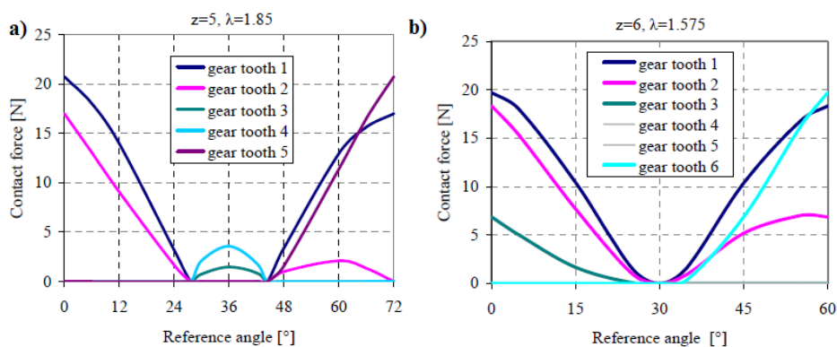
Slika 41. Usporedba kontaktnih sila kod parnog i neparnog broja zuba [16]
