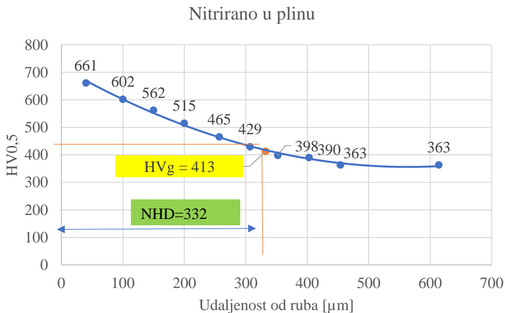
Sl. 61 Raspored mikrotvrdoće u plinski nitriranom sloju čelika 100Cr6 i određivanje efektivne dubine nitiranja
