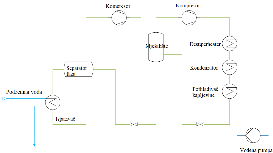
Slika 25. Shematski dijagram modelirane dizalice topline
