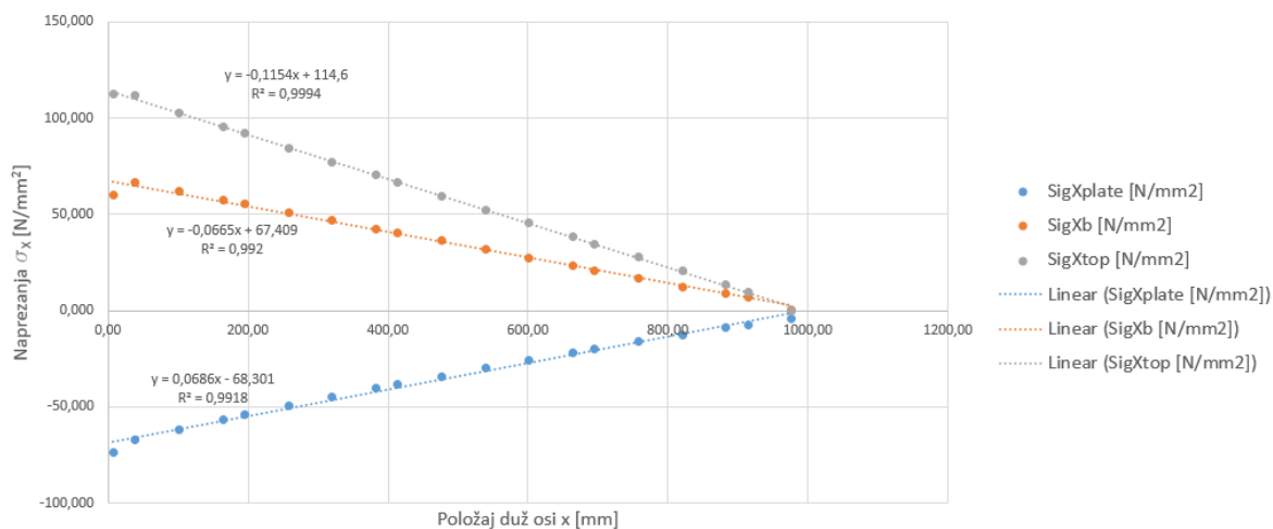
Slika 10. Grafički prikaz naprezanja \sigma_x duž grede s prikazanim interpolacijskim funkcijama za slučaj opterećenja 1
